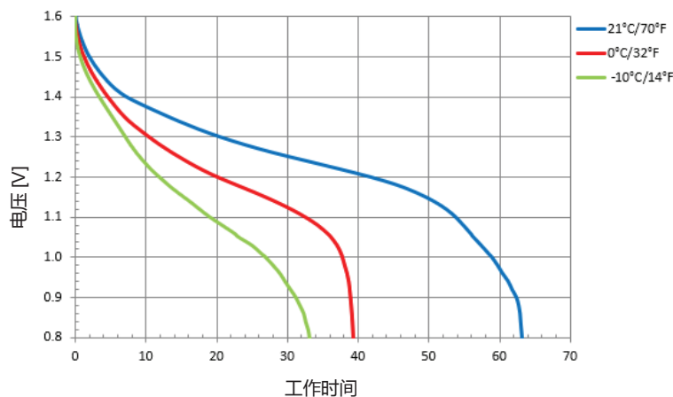
恒定电流 – 100mA
